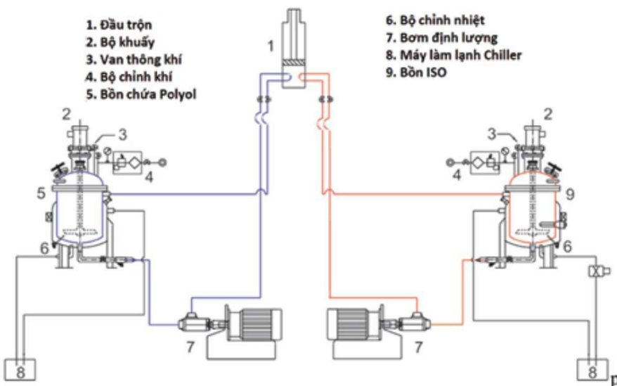
Nguyên lý hoạt động máy phun PU áp cao
